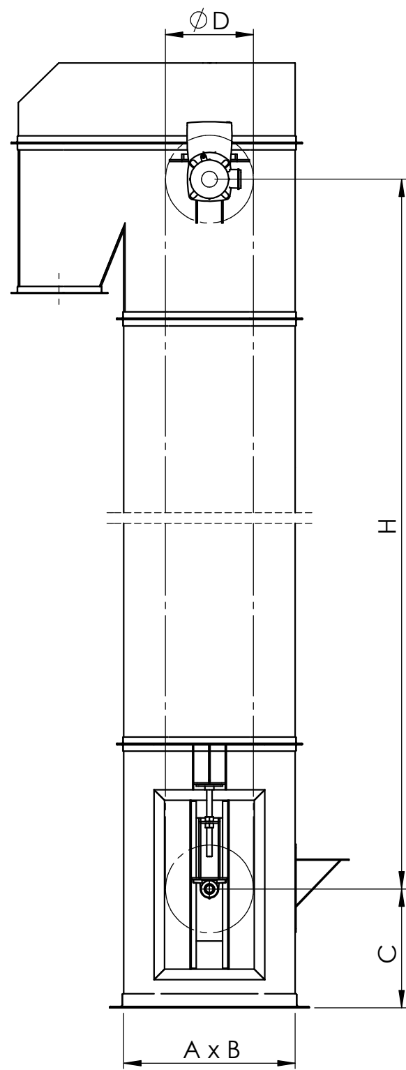
TPK - odśrodkowy
