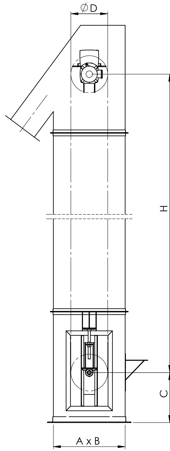
TPK - grawitacyjny
